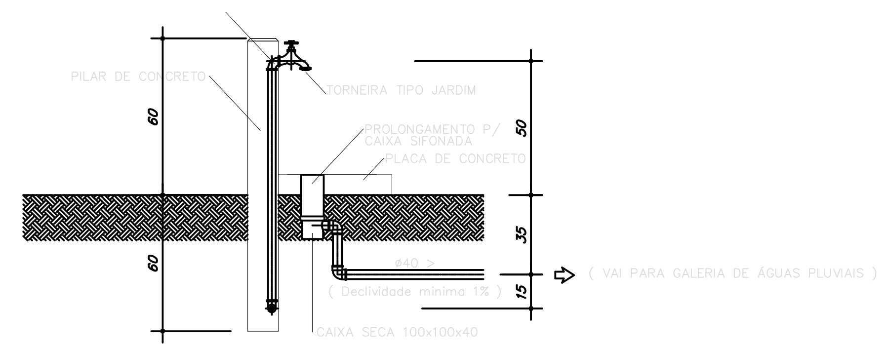
VISTA LATERAL PONTO DE ÁGUA EXTERNO Sem Escala
