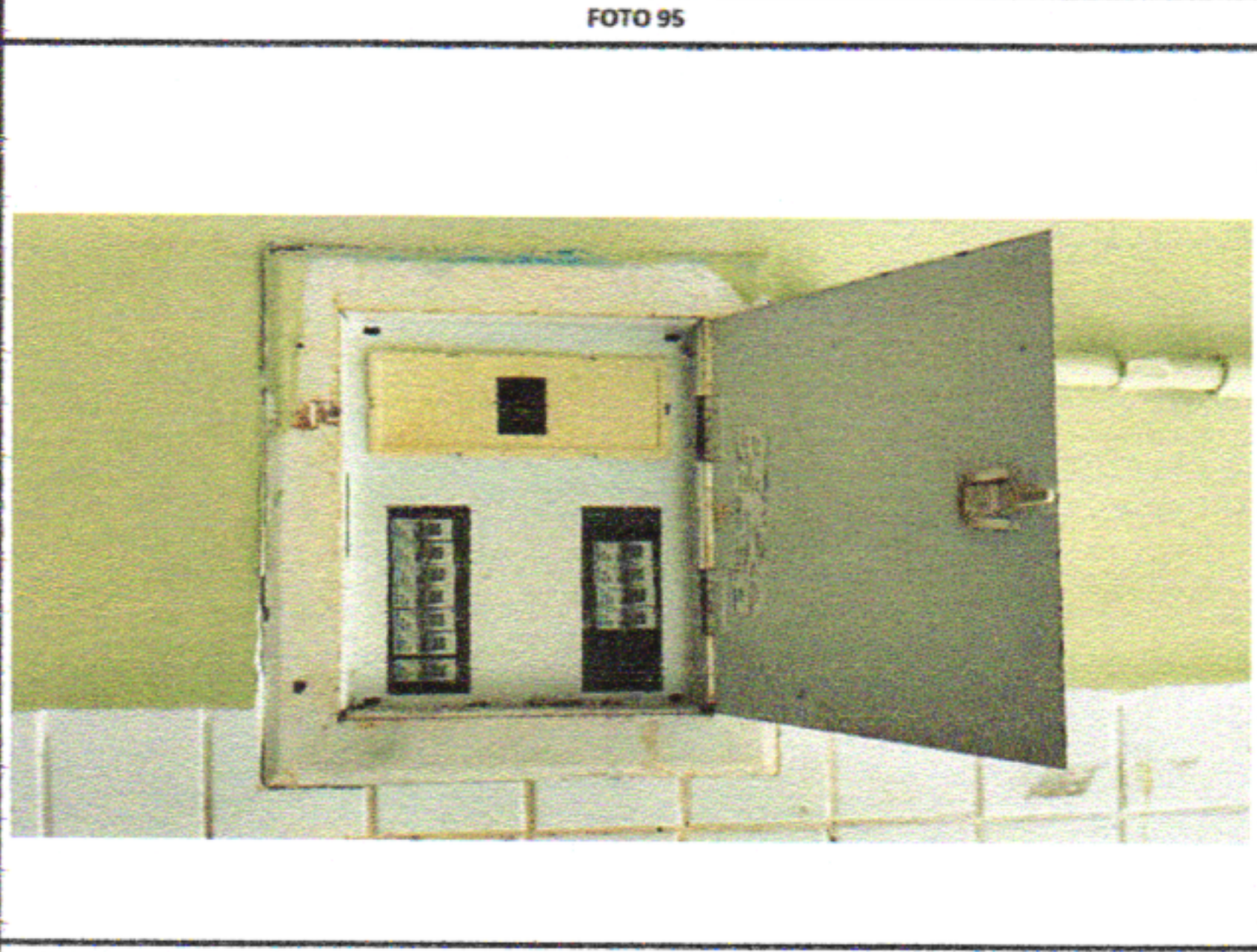
INSTALAÇÃO DE NOVOS DISJUNTORES MONOPOLAR DE 16A E 20A, E O DISJUNTOR GERAL DE 50A
