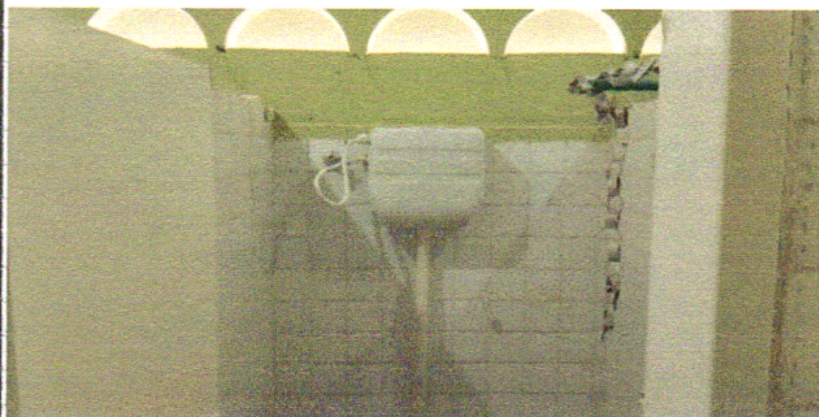
INSTALAÇÃO DA CAIXA DE DESCARGA DE SOBREPOR, ENGATE E KIT SALVA REGISTRO
