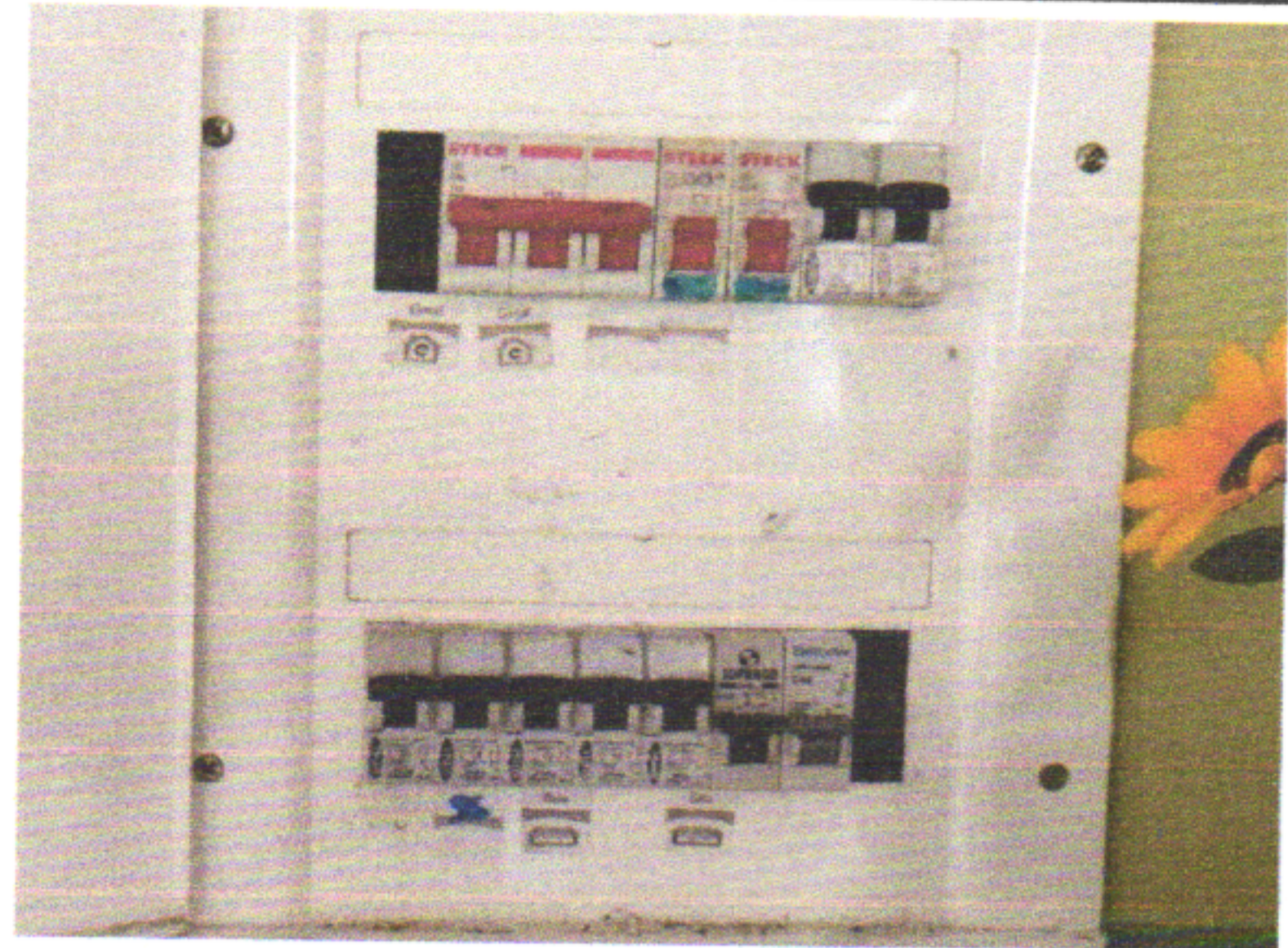
INSTALAÇÃO DE DISJUNTOR TRIPOLAR 50A E DISJUNTOR MONOPOLAR 40A NO QUADRO DE DISTRIBUIÇÃO
