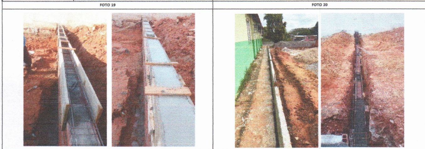
ESCOLA MUNICIPAL ERCINA LAPENDA - BASE DA QUADRA (ALVENARIA E CINTA)
