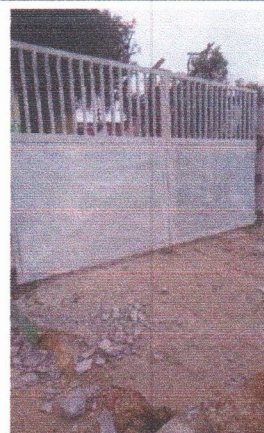
ESCOLA MUNICIPAL ERCINA LAPENDA - PORTÃO DE ENTRADA EM FERRO DUAS FOLHAS (PORTÃO VEÍCULOS)
