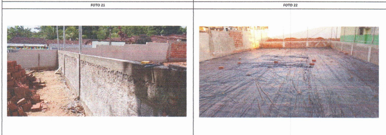
ESCOLA MUNICIPAL ERCINA LAPENDA - MURETA DA QUADRA (ALVENARIA, PILARES, BALDRAME E CINTA)
